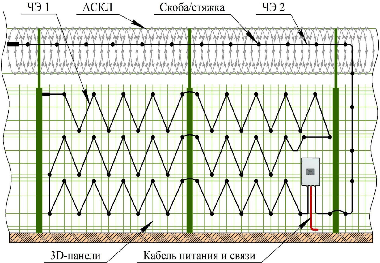
Рисунок А.1 – Конфигурация зон обнаружения вариант 1
