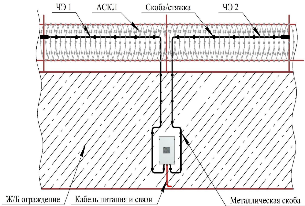
Рисунок А.2 – Конфигурация зон обнаружения вариант 2
